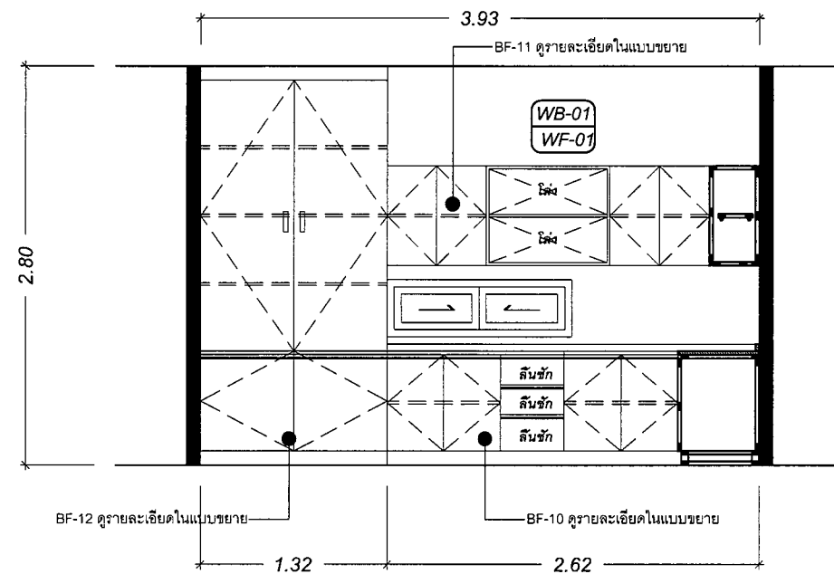
ELEVATION : A
