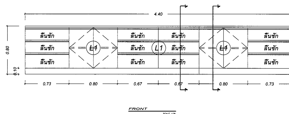
แบบขยาย BF-03
