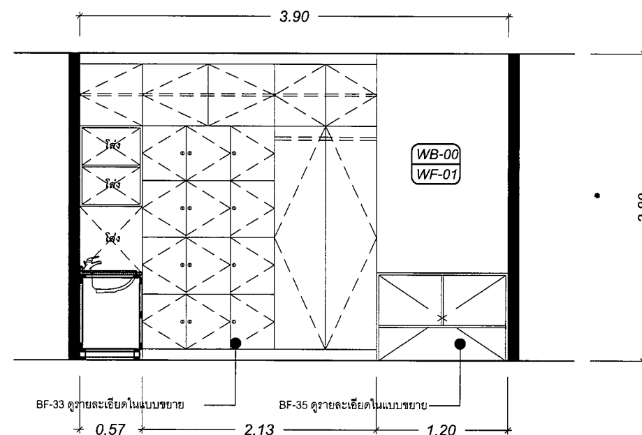
ELEVATION : D
