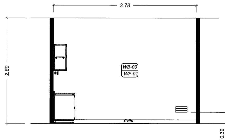
ELEVATION : C
