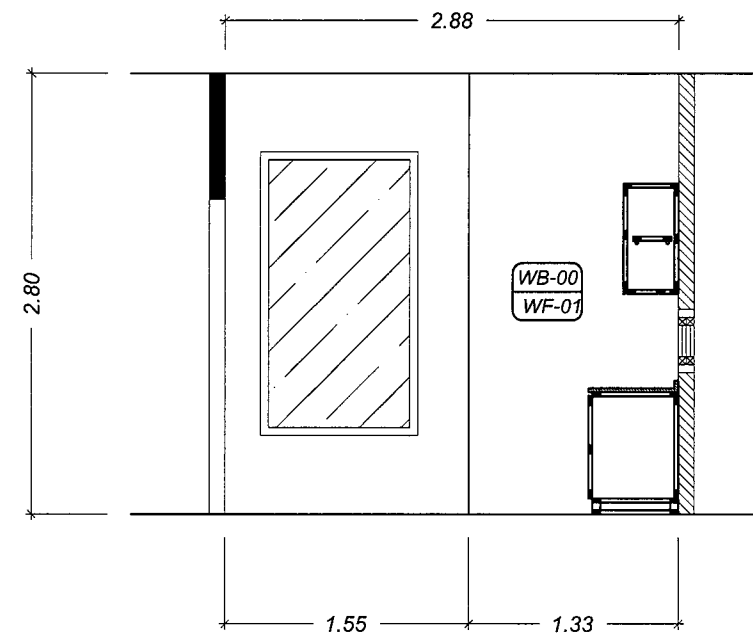
ELEVATION : C
