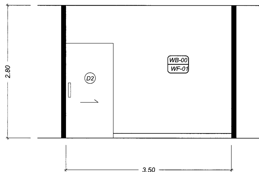
ELEVATION : B
