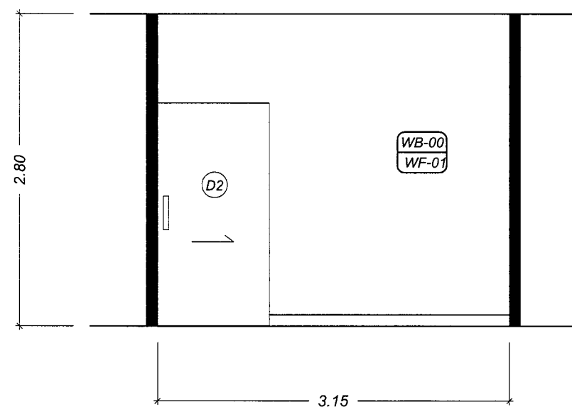
ELEVATION : B
