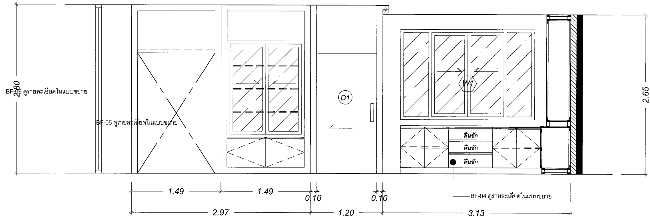
ELEVATION : D
