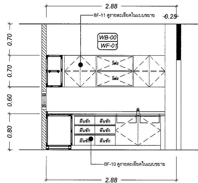
ELEVATION : D
