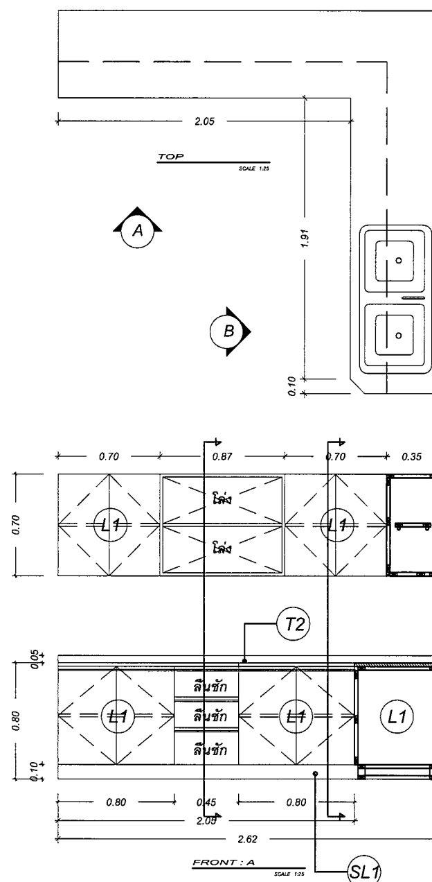
แบบขยาย BF-10 : BF-11
