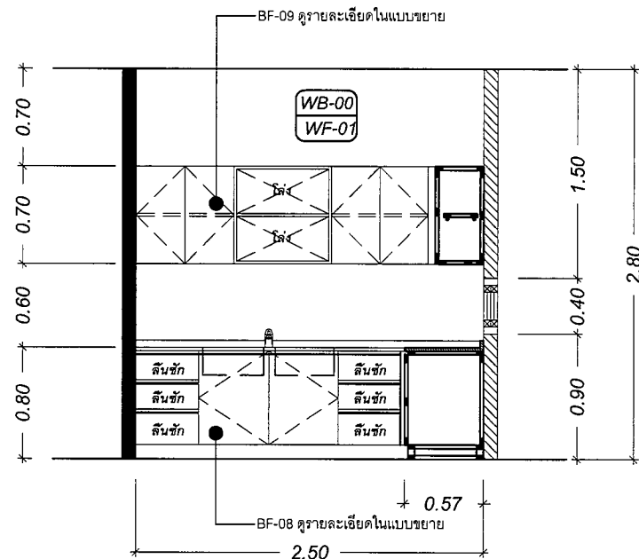
ELEVATION : D
