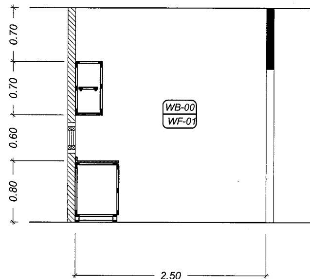
ELEVATION : C
