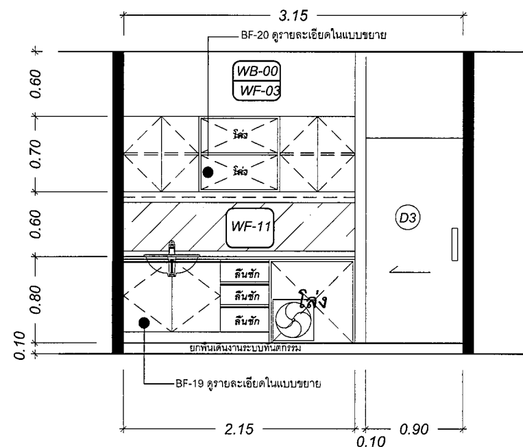
ELEVATION : A
