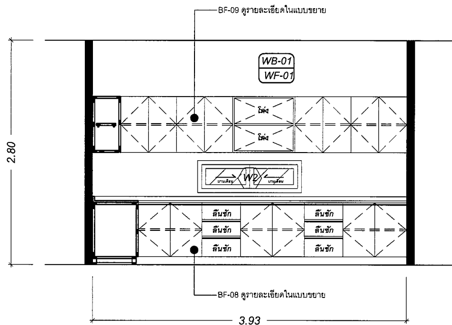
ELEVATION : A
