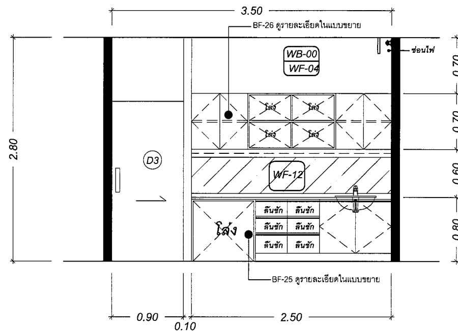
ELEVATION : A
