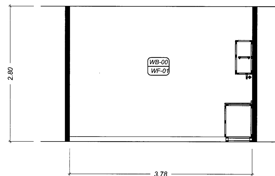
ELEVATION : D
