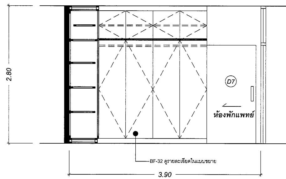
ELEVATION : D
