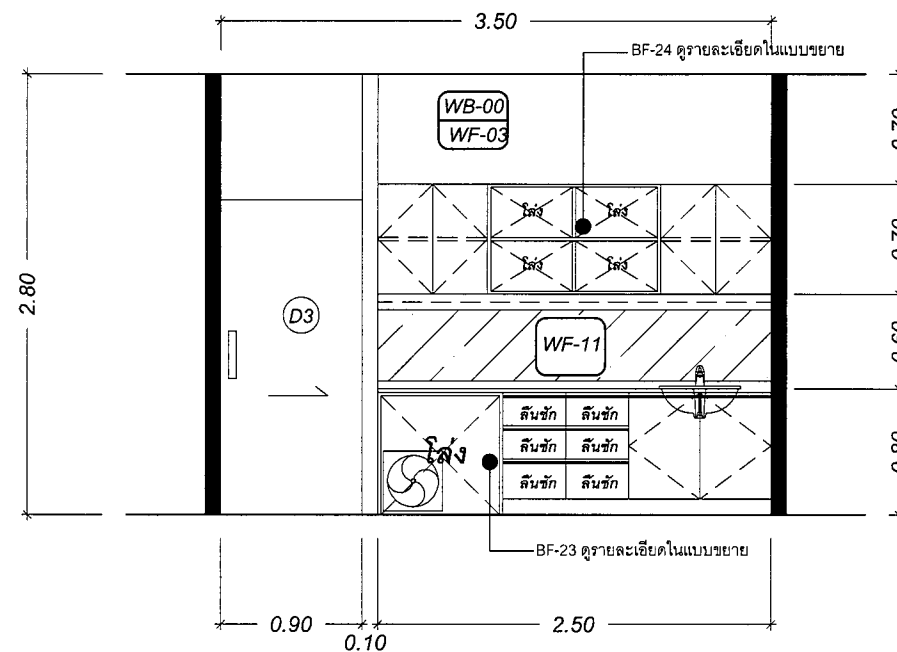
ELEVATION : A
