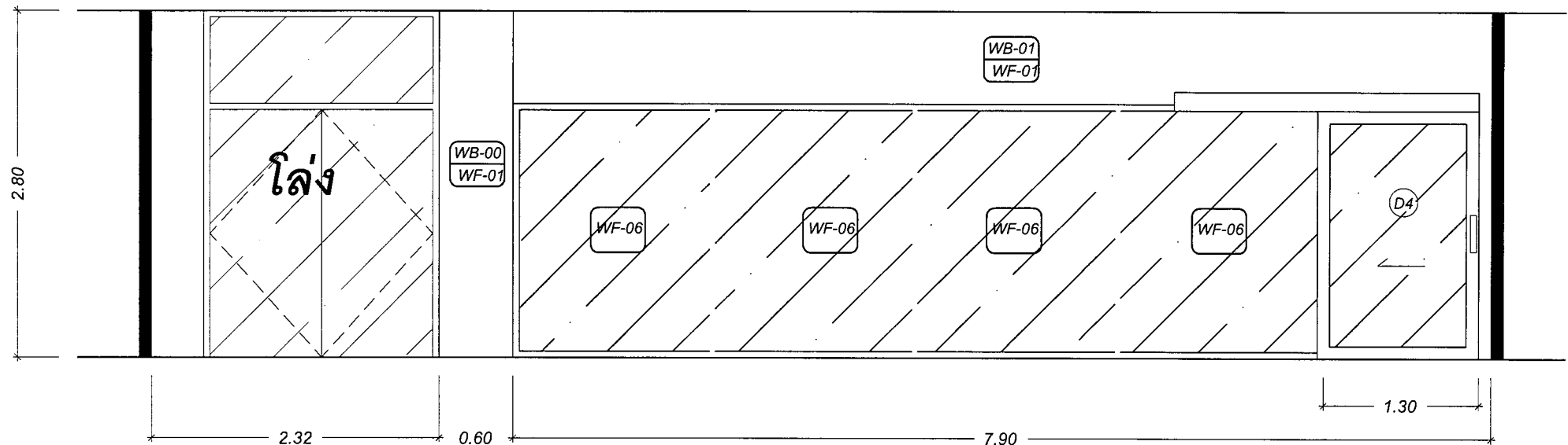
ELEVATION : F
