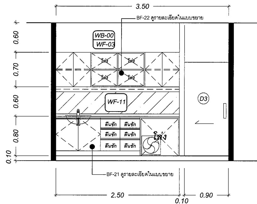
ELEVATION : A
