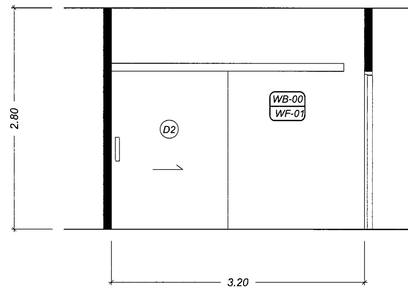
ELEVATION : B
