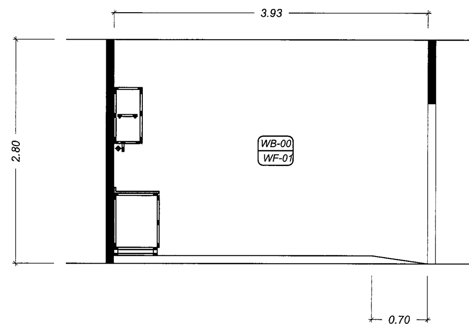
ELEVATION : C
