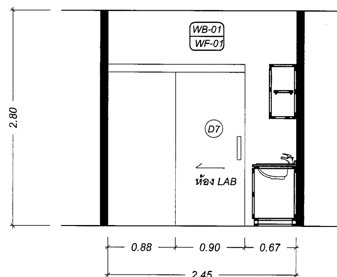
ELEVATION : D
