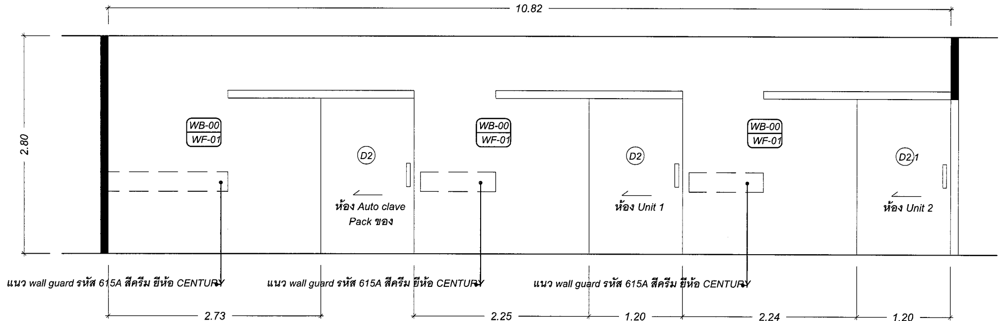
ELEVATION : G
