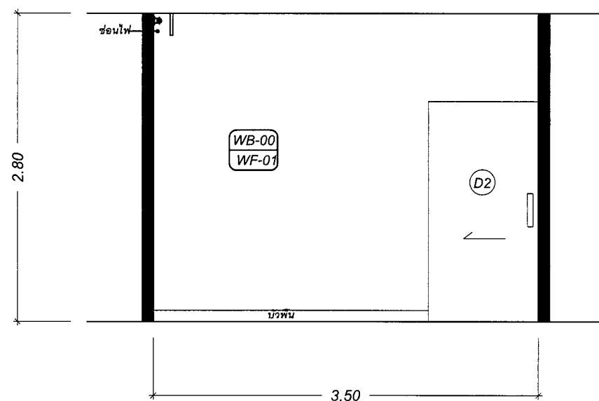
ELEVATION : B
