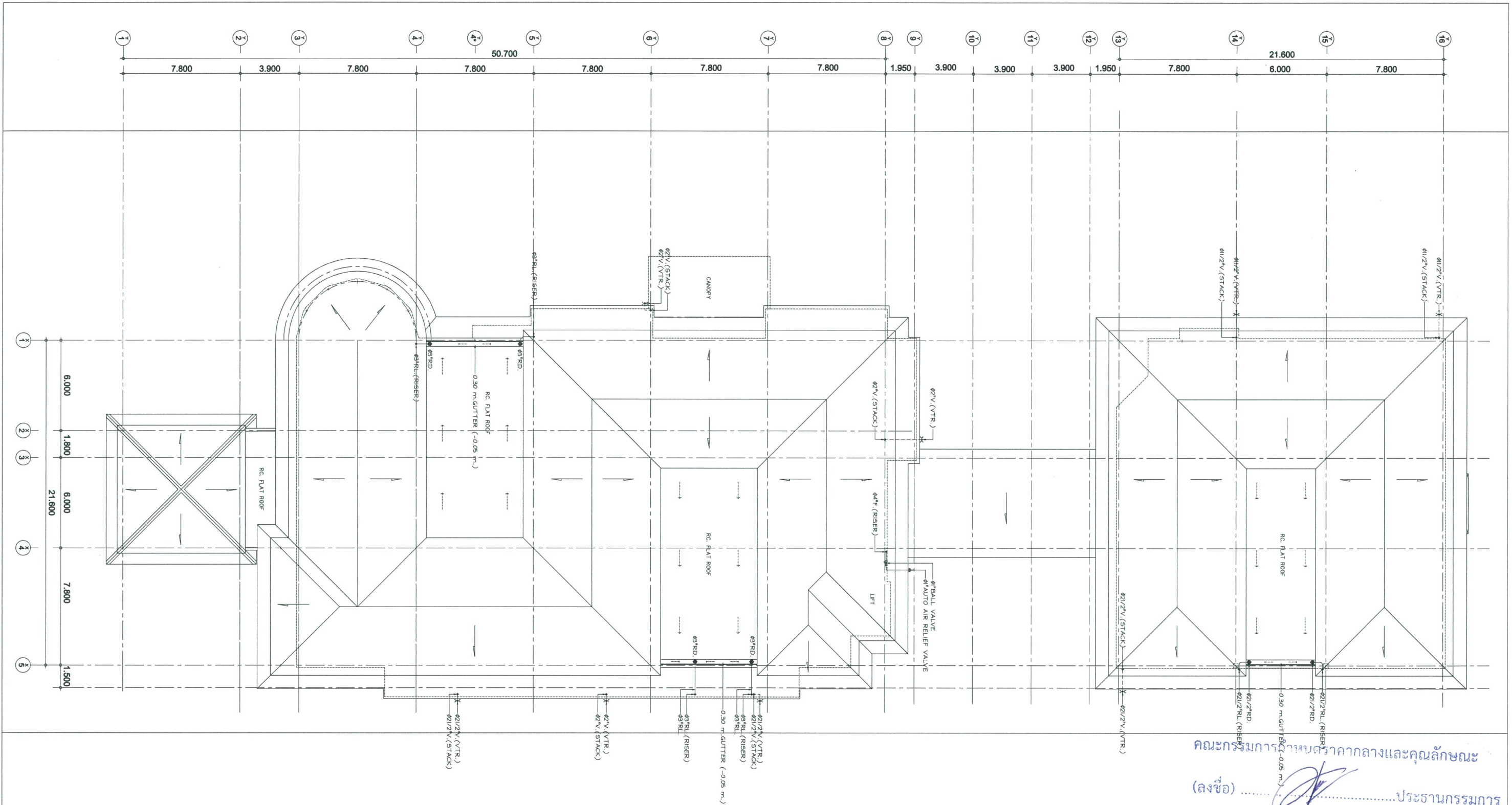
แปลนระบบวิศวกรรมสิ่งแวดล้อมพื้นที่หลังคา Scale 1 : 125
